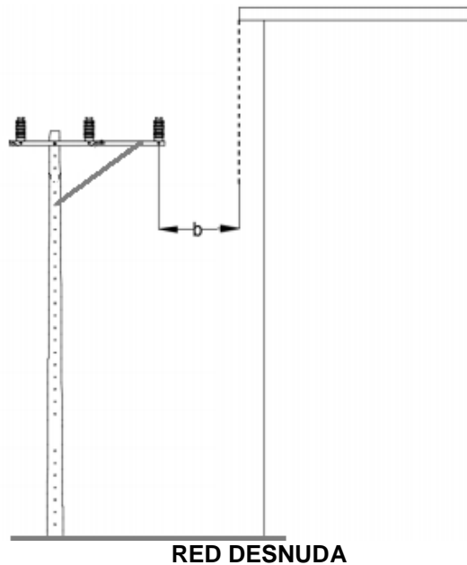
Figura 4. Distancia horizontal entre la red eléctrica con conductores desnudos y la proyección de una edificación por encima de la red, caso B.
