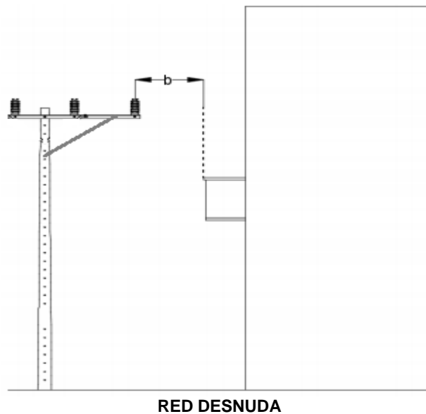
Figura 2. Distancia horizontal entre la red eléctrica con conductores desnudos y la proyección de una edificación por debajo de la red, caso B.
