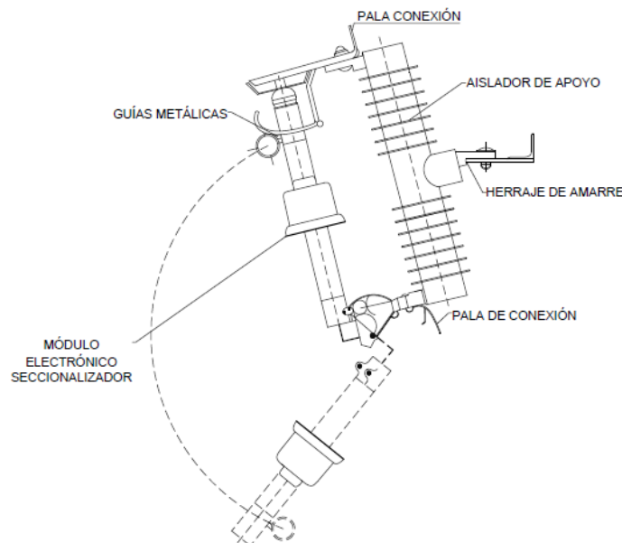
Figura 12. Seccionalizador electrónico
