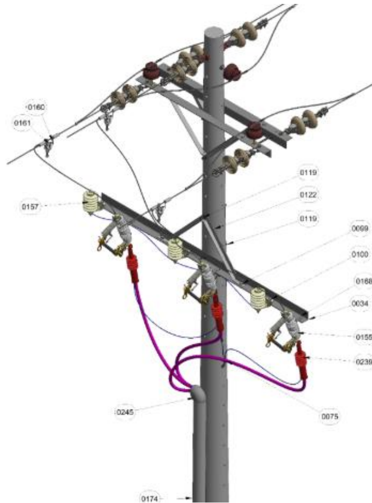
Figura 17. Transición de red aérea desnuda a subterránea
