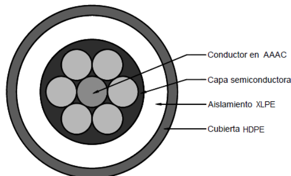
Figura 7. Cable cubierto de tres capas
